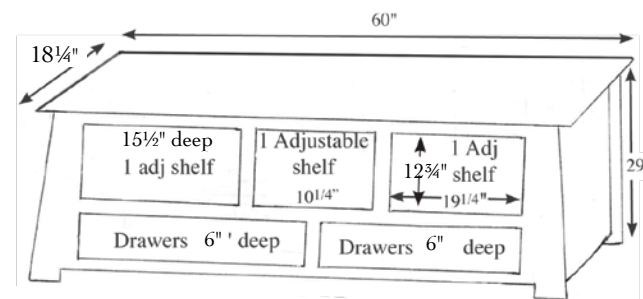
FVE-032-CN-BP FVE-032-CB-BP (top size = 18 3/4 D x 61 1/4 W) FVE-032-MD-BP; FVE-032-WL-BP
